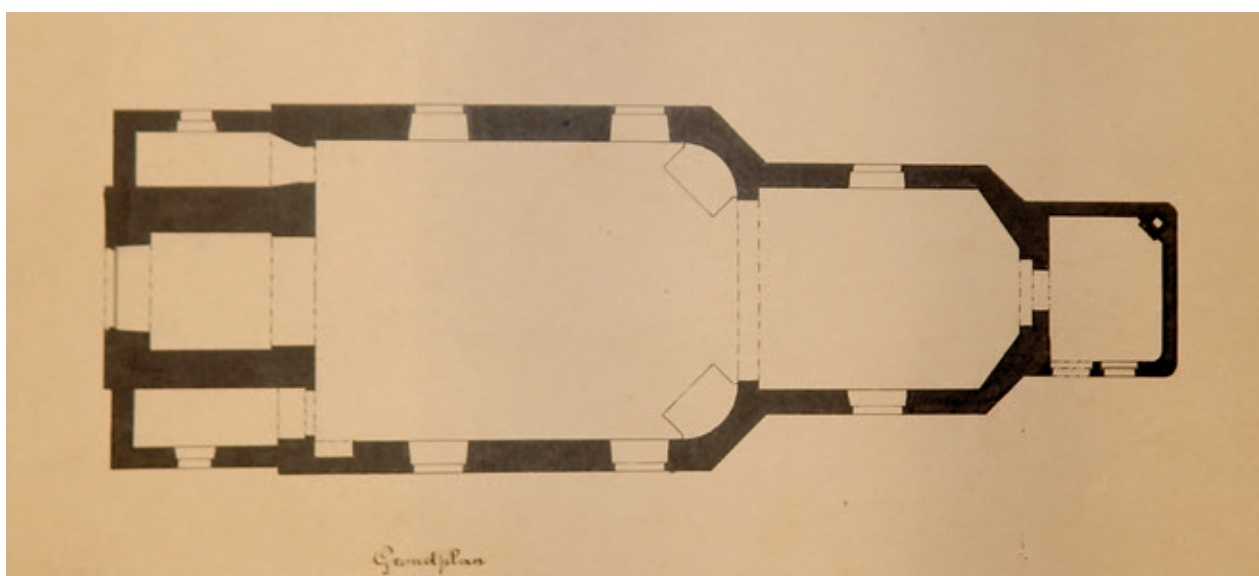
Zijaanzicht en grondplan van de kerk zoals Christiaens ze in 1895 aantrof
